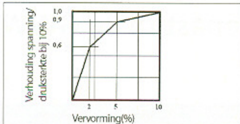
↑ Figuur 1 Spannings/rekdiagram
